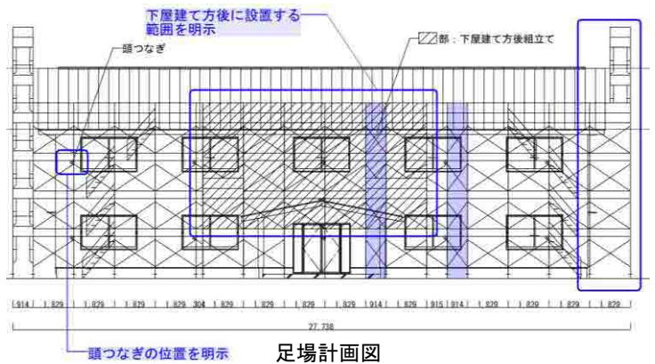
足場計画図
