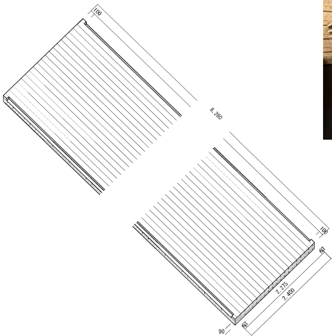
CLTパネル 1枚 (3層3プライ)
